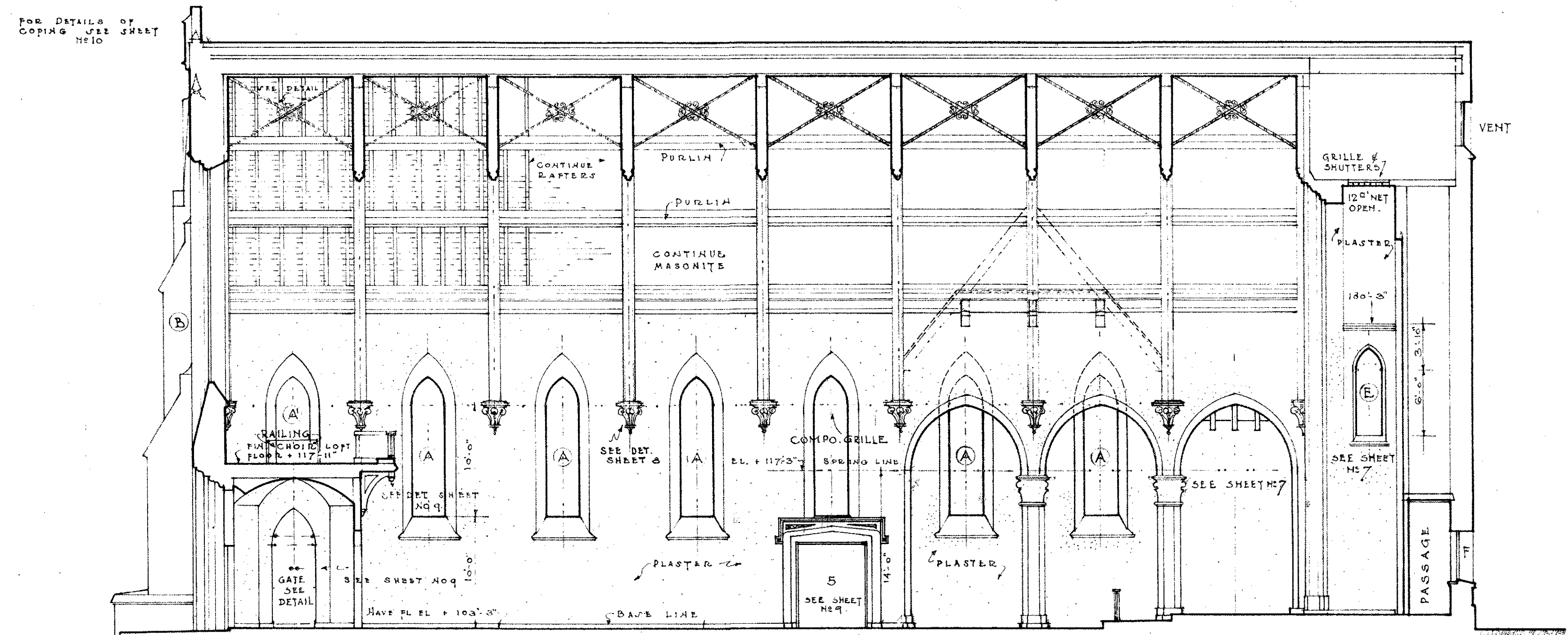
LONGITUDINAL SECTION
